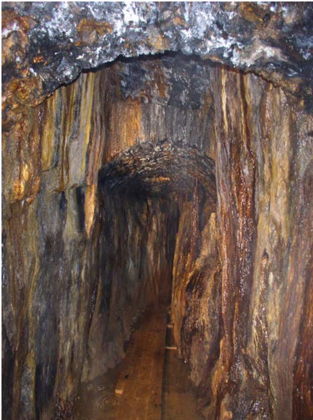
Hauptstollengang auf der 1. Sohle der „Reichen Zeche“ (Foto Tondera)
